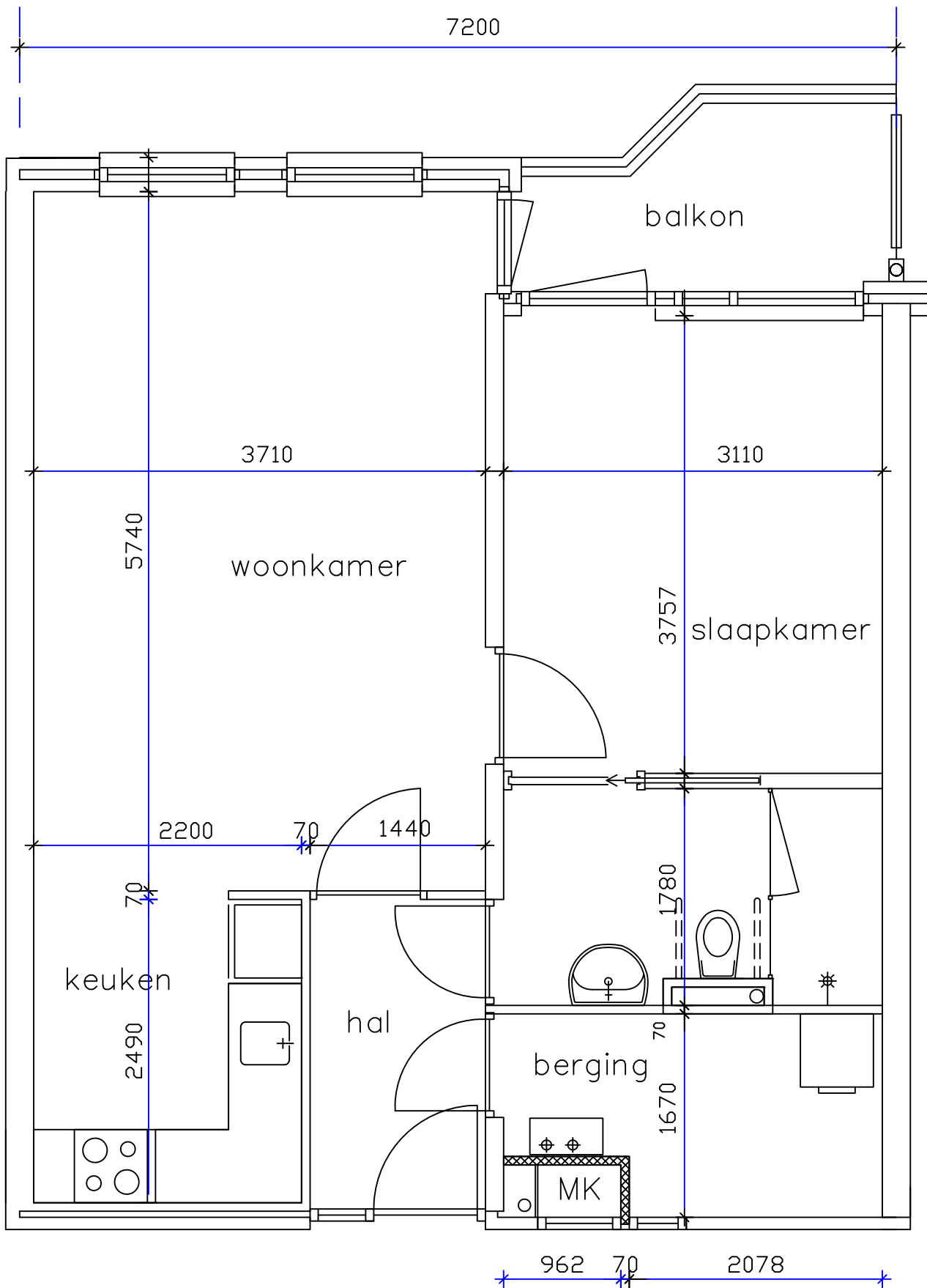
2 kamer appartement Kerkstraat maatvoeringen zijn indicatiematen
